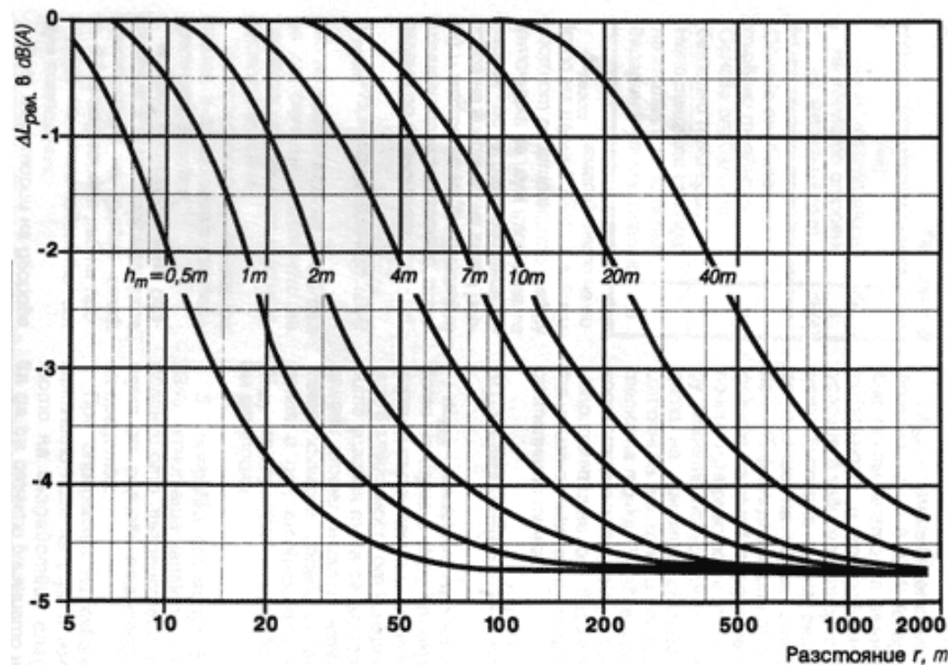
Фиг.1.4. Определяне на D_{L_{\text{рел.}}} - намаляване на нивото на шума в dB(A) в зависимост от средната височина h_m на разпространение на шума и разстоянието r между източника на шум и изчислителната точка
