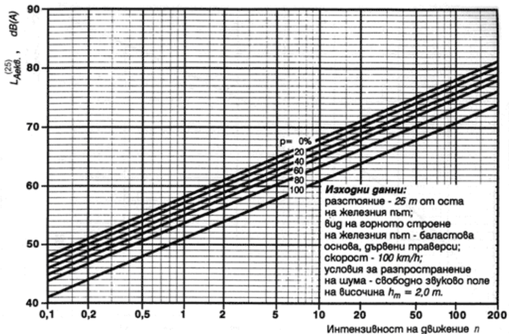
Фиг.2.1. L_{\text{Аекв.Т(25m)}} - еквивалентно ниво на шума в dB(A), в зависимост от средния брой влакови композиции за час n и брой вагони с дискови спирачки p в %.
