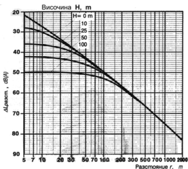
Фиг. 4.1. Определяне на D_{L\text{разст.}} - намаляване на нивото на шума в dB(A) в
