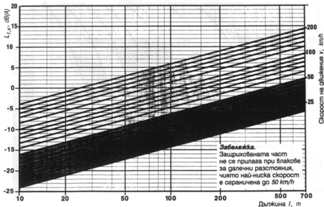
Фиг.2.2. Определяне на D_{Ll,v} - поправка в dB(A), за различни скорости на движение v в зависимост от дължината l на влаковата композиция
