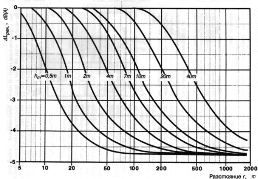
Фиг. 2.4. Определяне на D_{L\text{рел}} - намаляване на нивото на шума в dB(A) в зависимост от средната височина h_m на разпространение на шума и разстоянието r между източника на шум и изчислителната точка.
